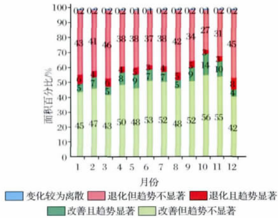
图 2 月尺度 NDVI 变化特征对比
