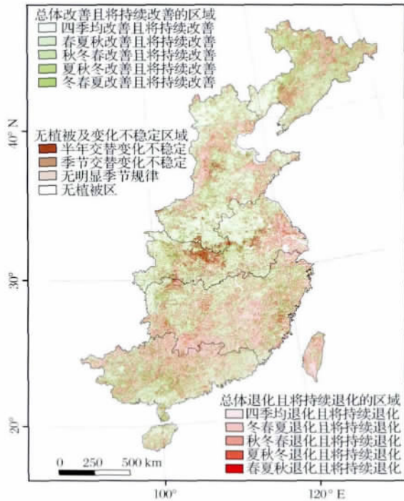
图 4 NDVI 的季节演化态势图谱
