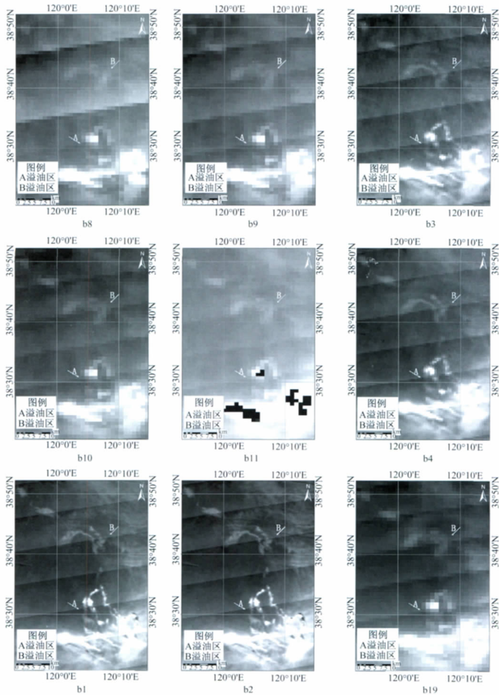
图6 2011年MODIS单波段影像
