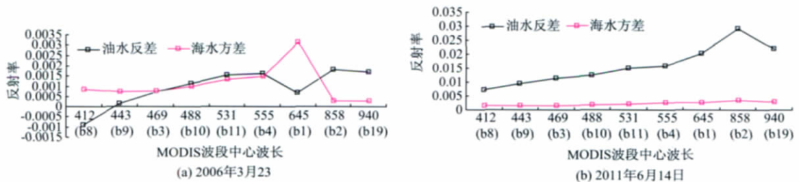
图4 油水反差及海水方差曲线
