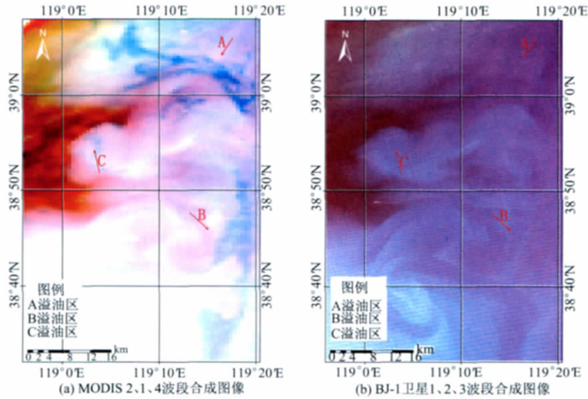
图2 不同卫星的假彩色合成影像 Fig. 2 Different satellite false color image
