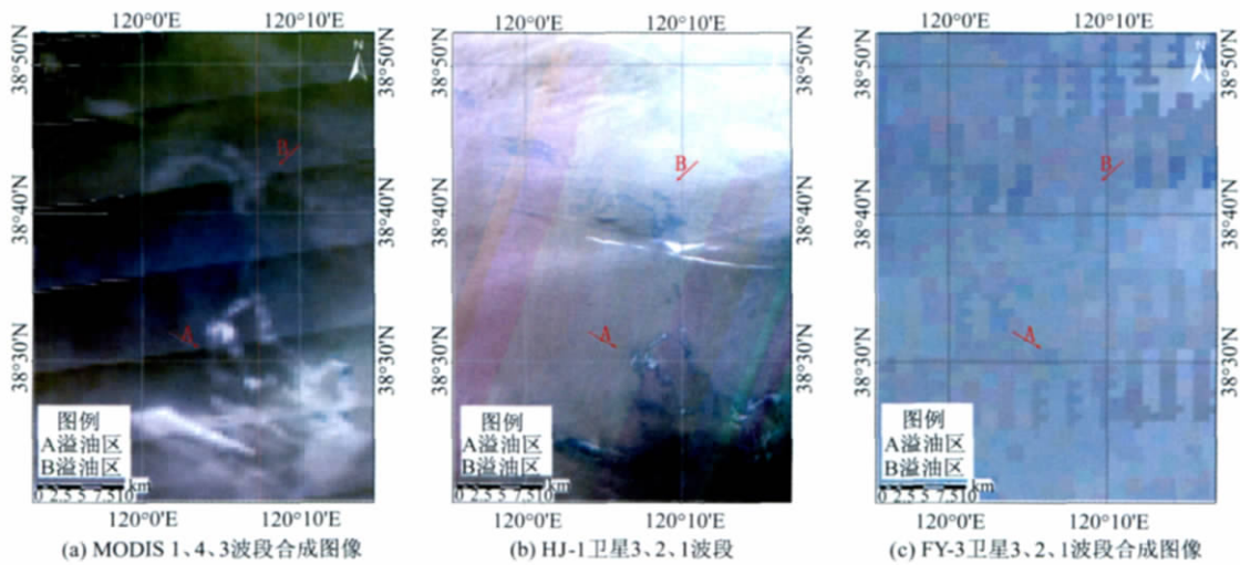
图3 不同卫星的真彩色合成影像 Fig. 3 Different satellite true color image
