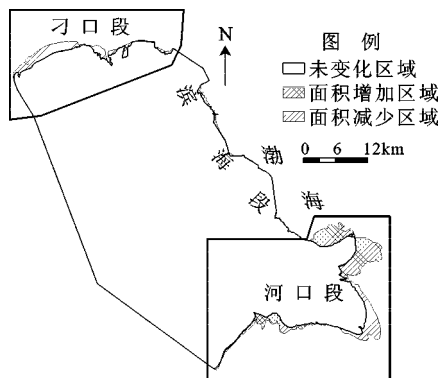
图3 黄河三角洲海岸线和陆地变迁
