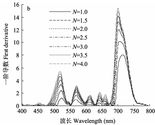
图 1 不同叶肉结构参数 N 条件下模拟的叶片光谱(a)和一阶导数(b)
