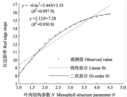
图 2 叶肉结构参数 N 和红边斜率的关系
