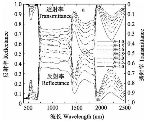
图 1 不同叶肉结构参数 N 条件下模拟的叶片光谱(a)和一阶导数(b)
